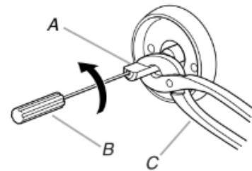
A. Vástago de la perilla de control
