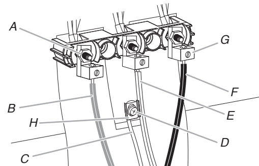
A. Écrou hexagonal 10 – 32 B. Ligne 2 (rouge) C. Fil de mise à la terre nu (vert) D. Vis de liaison à la terre E. Conducteur du neutre (blanc) F. Ligne 1 (noir) G. Cosse H. Embout de la barrette de liaison à la terre
