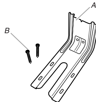
A. Bride antibascullement B. 2 vis no 12 x 1 5/8 po (4,1 cm)
